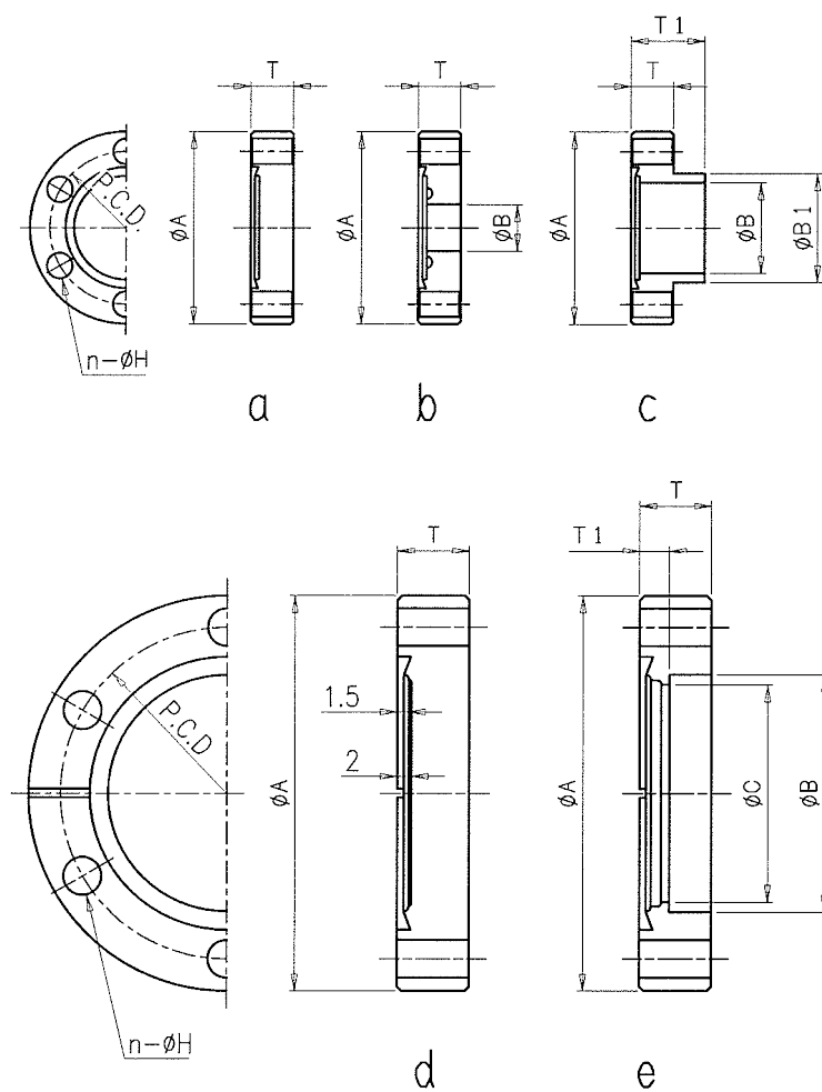
第4図 ICF 固定フランジの形状
