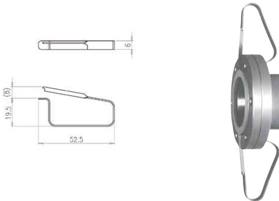
第 8 図 ガスケットクリップの形状と使用例
