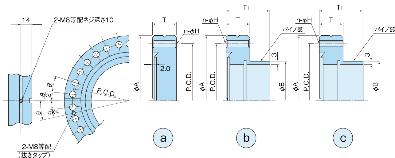
第 6 図 大口径 ICF 固定フランジの形状
